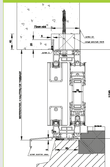
Dormant de 70 mm
