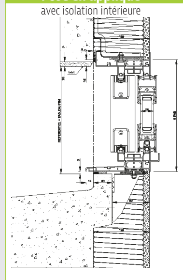
Possibilité de dormant monobloc 100/120/140/160 mm
